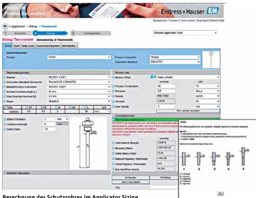
Berechnung des Schutzrohres im Applicator Sizing
